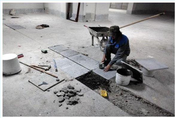
اجرای لکه گیری سنگ کف پارکینگ منفی یک
